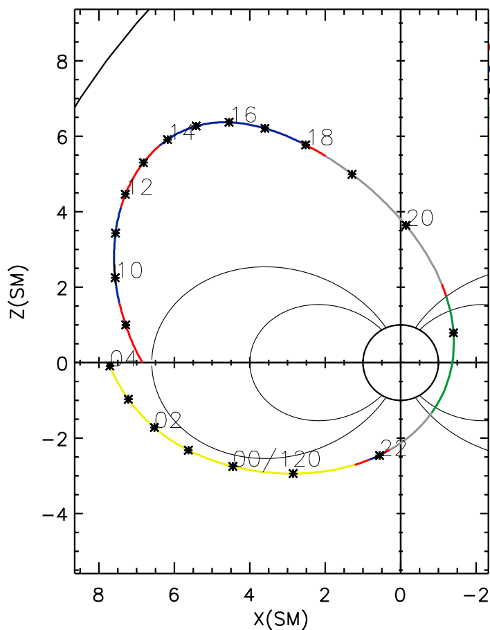
POLAR orbit 2001 119 (04/29) 08:12 UT to 2001 120 (04/30) 04:03 UT
