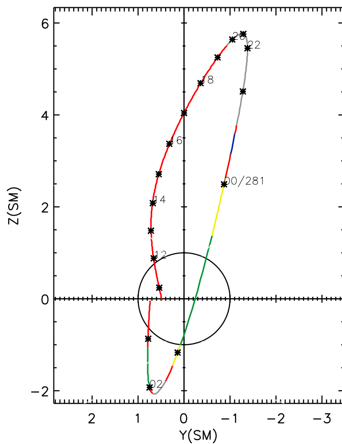
POLAR orbit 2000 280 (10/06) 10:36 UT to 2000 281 (10/07) 03:39 UT
