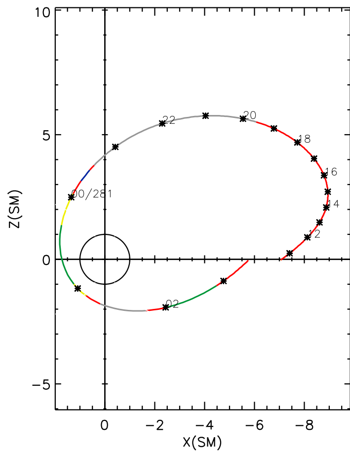
POLAR orbit 2000 280 (10/06) 10:36 UT to 2000 281 (10/07) 03:39 UT
