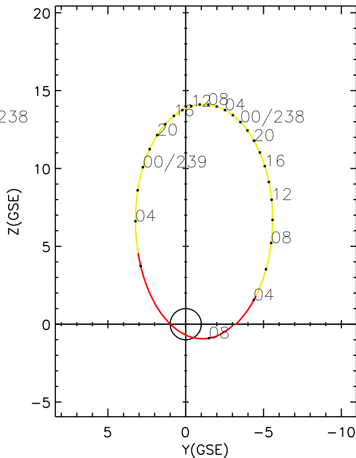
CLUSTER 2 orbit 2024 237 (08/24) 02:36 UT to 2024 239 (08/26) 08:46 UT
