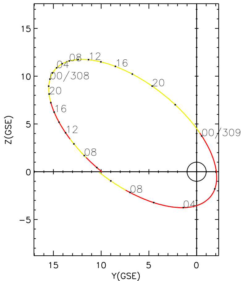
CLUSTER 2 orbit 2022 307 (11/03) 05:16 UT to 2022 309 (11/05) 11:26 UT
