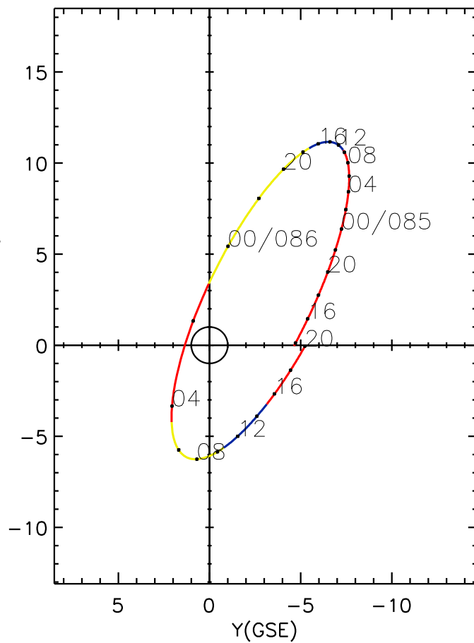
CLUSTER 2 orbit 2021 084 (03/25) 13:46 UT to 2021 086 (03/27) 20:01 UT
