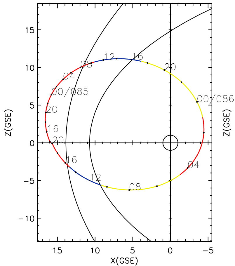
CLUSTER 2 orbit 2021 084 (03/25) 13:46 UT to 2021 086 (03/27) 20:01 UT
