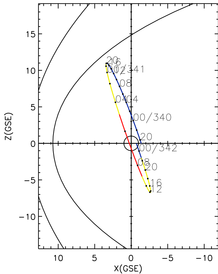
CLUSTER 2 orbit 2020 339 (12/04) 19:16 UT to 2020 342 (12/07) 01:31 UT
