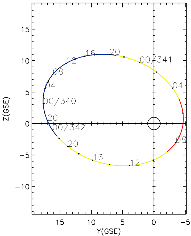
CLUSTER 2 orbit 2020 339 (12/04) 19:16 UT to 2020 342 (12/07) 01:31 UT
