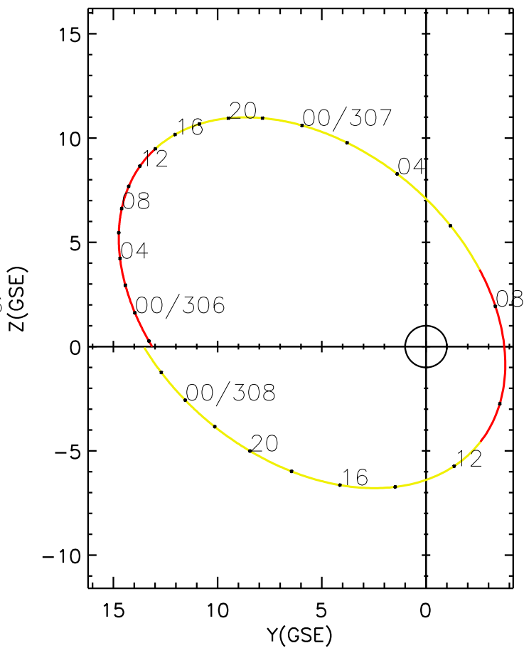
CLUSTER 2 orbit 2020 305 (10/31) 21:36 UT to 2020 308 (11/03) 03:46 UT
