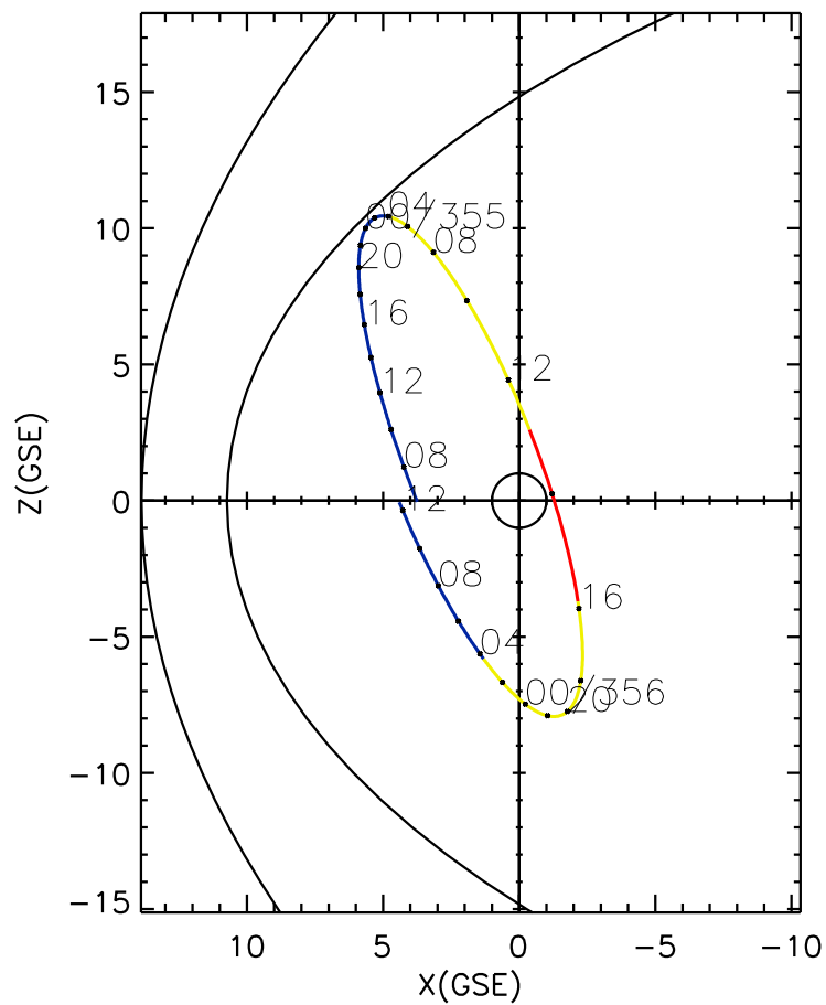
CLUSTER 2 orbit 2019 354 (12/20) 06:11 UT to 2019 356 (12/22) 12:26 UT
