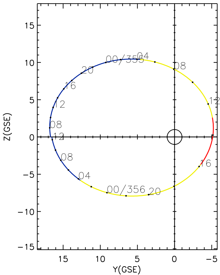
CLUSTER 2 orbit 2019 354 (12/20) 06:11 UT to 2019 356 (12/22) 12:26 UT
