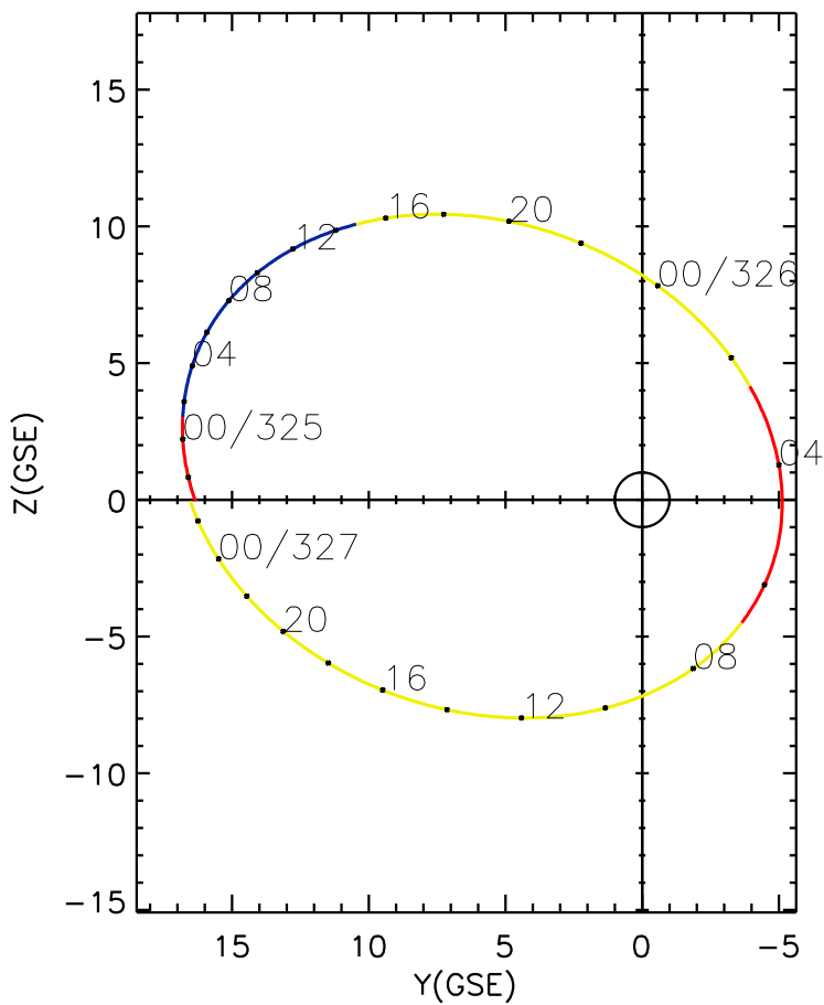
CLUSTER 2 orbit 2019 324 (11/20) 20:46 UT to 2019 327 (11/23) 03:01 UT
