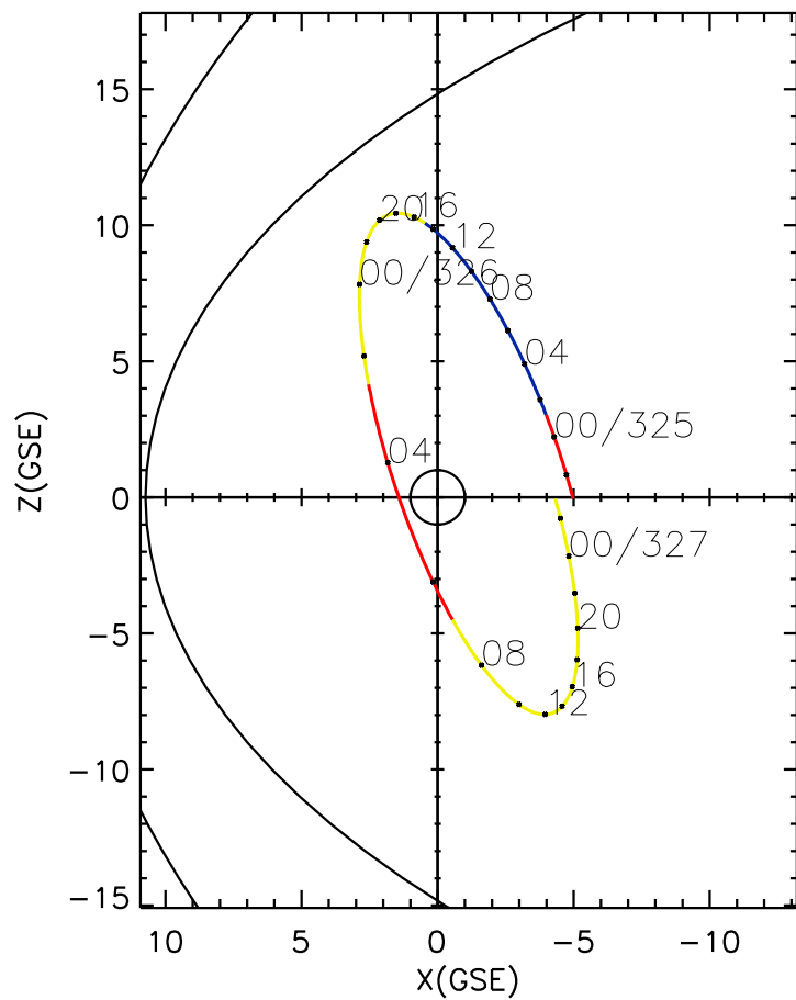
CLUSTER 2 orbit 2019 324 (11/20) 20:46 UT to 2019 327 (11/23) 03:01 UT
