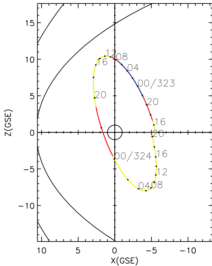
CLUSTER 2 orbit 2019 322 (11/18) 14:31 UT to 2019 324 (11/20) 20:46 UT
