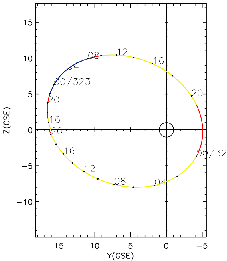
CLUSTER 2 orbit 2019 322 (11/18) 14:31 UT to 2019 324 (11/20) 20:46 UT
