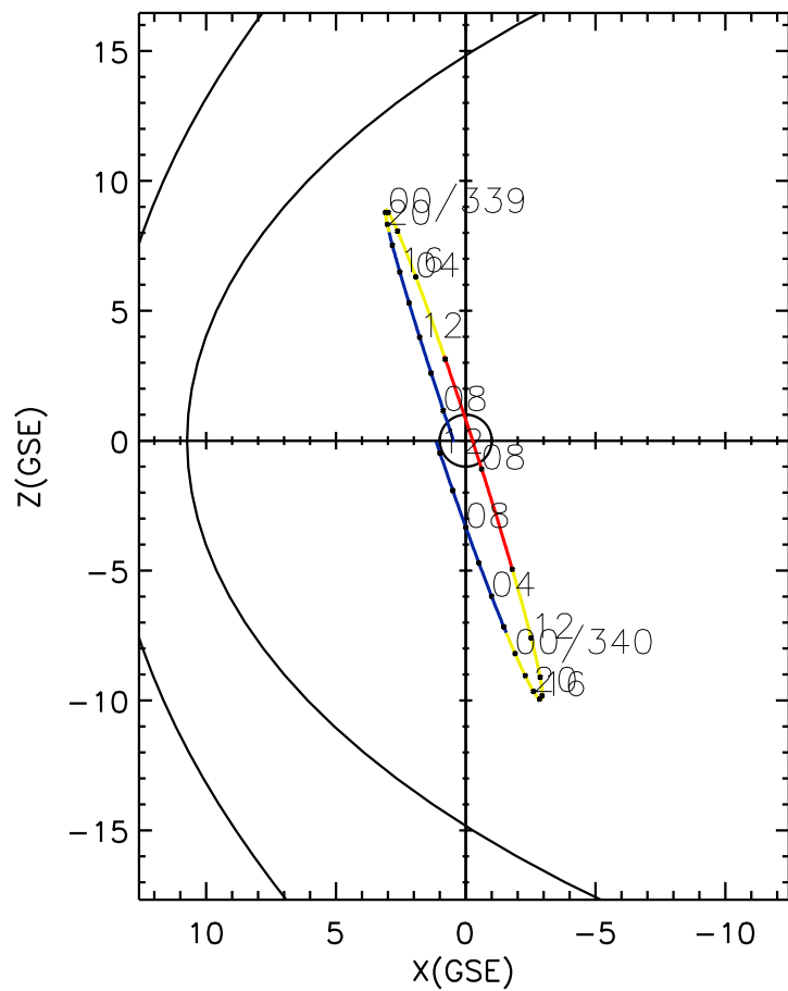
CLUSTER 2 orbit 2017 338 (12/04) 06:21 UT to 2017 340 (12/06) 12:36 UT
