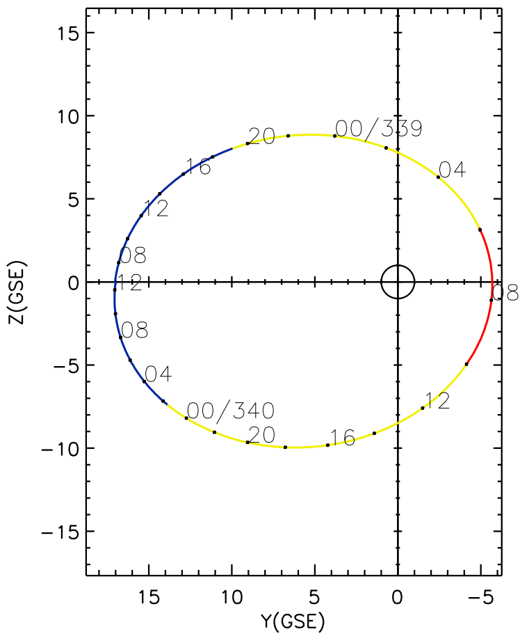
CLUSTER 2 orbit 2017 338 (12/04) 06:21 UT to 2017 340 (12/06) 12:36 UT
