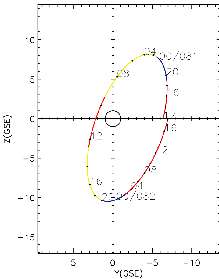
CLUSTER 2 orbit 2017 080 (03/21) 11:56 UT to 2017 082 (03/23) 18:11 UT
