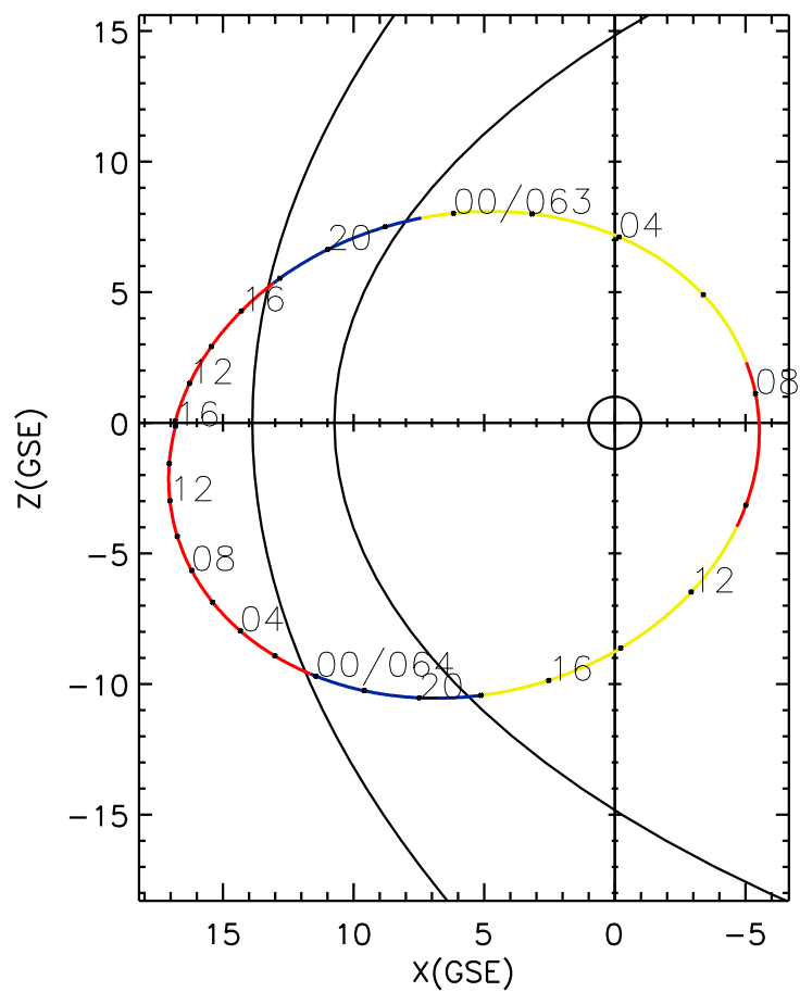
CLUSTER 2 orbit 2017 062 (03/03) 09:51 UT to 2017 064 (03/05) 16:06 UT
