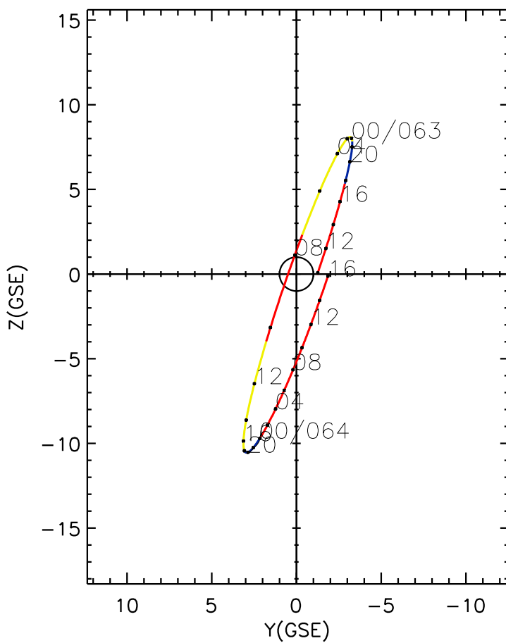
CLUSTER 2 orbit 2017 062 (03/03) 09:51 UT to 2017 064 (03/05) 16:06 UT
