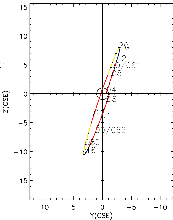
CLUSTER 2 orbit 2017 060 (03/01) 03:36 UT to 2017 062 (03/03) 09:51 UT
