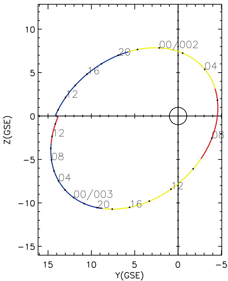
CLUSTER 2 orbit 2017 001 (01/01) 08:56 UT to 2017 003 (01/03) 15:11 UT
