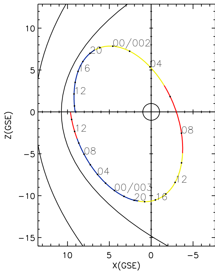
CLUSTER 2 orbit 2017 001 (01/01) 08:56 UT to 2017 003 (01/03) 15:11 UT
