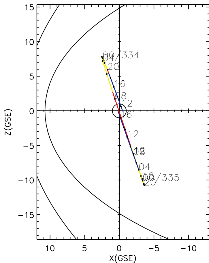
CLUSTER 2 orbit 2016 333 (11/28) 11:01 UT to 2016 335 (11/30) 17:21 UT
