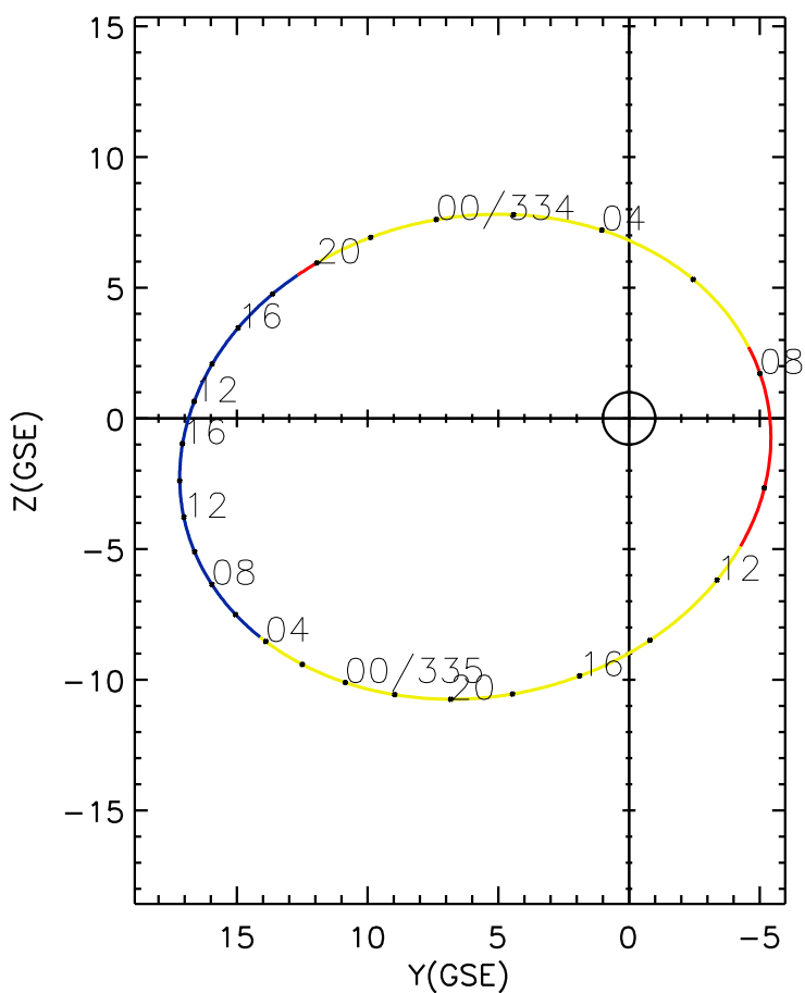
CLUSTER 2 orbit 2016 333 (11/28) 11:01 UT to 2016 335 (11/30) 17:21 UT
