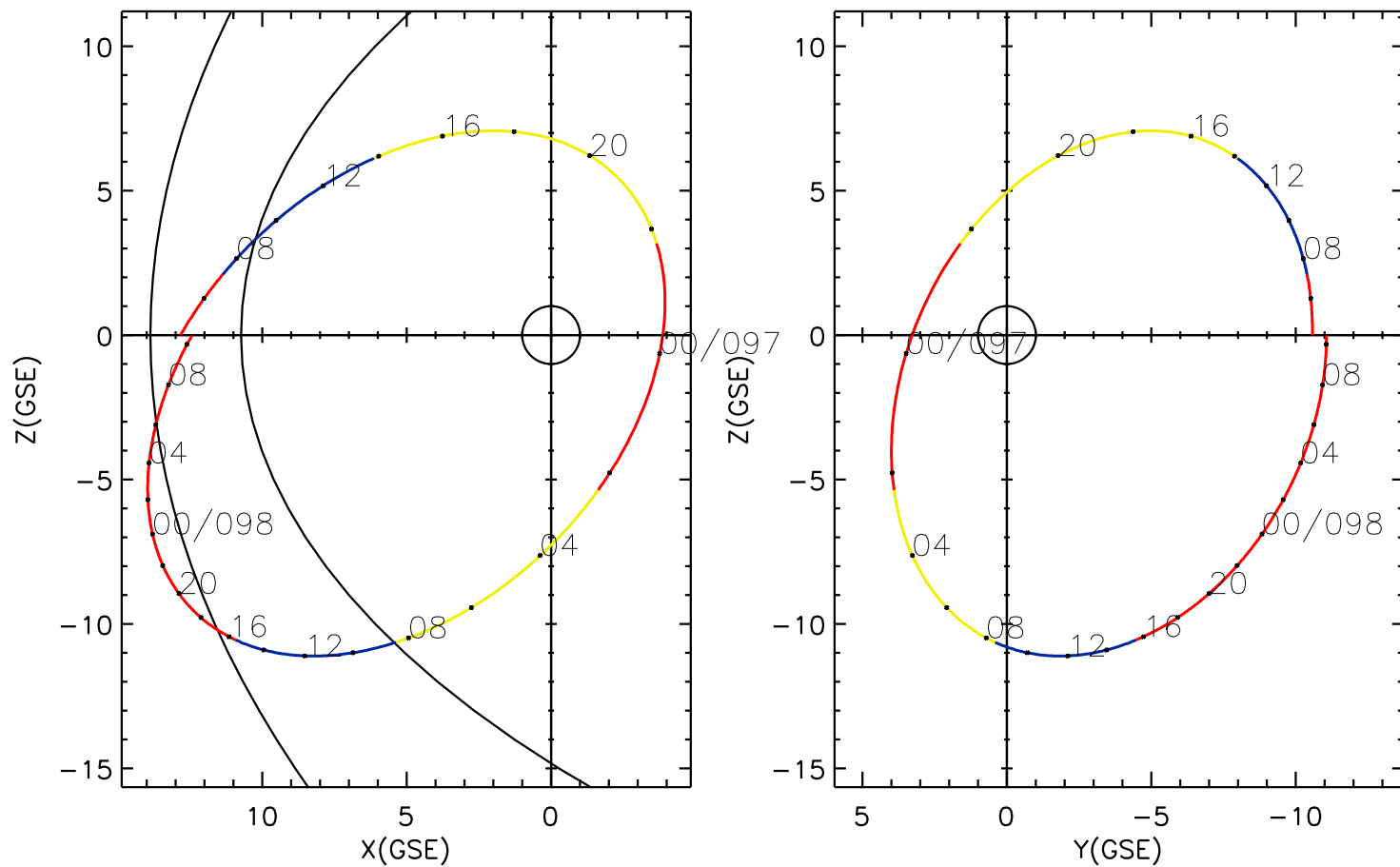
CLUSTER 2 orbit 2016 096 (04/05) 04:11 UT to 2016 098 (04/07) 10:26 UT
