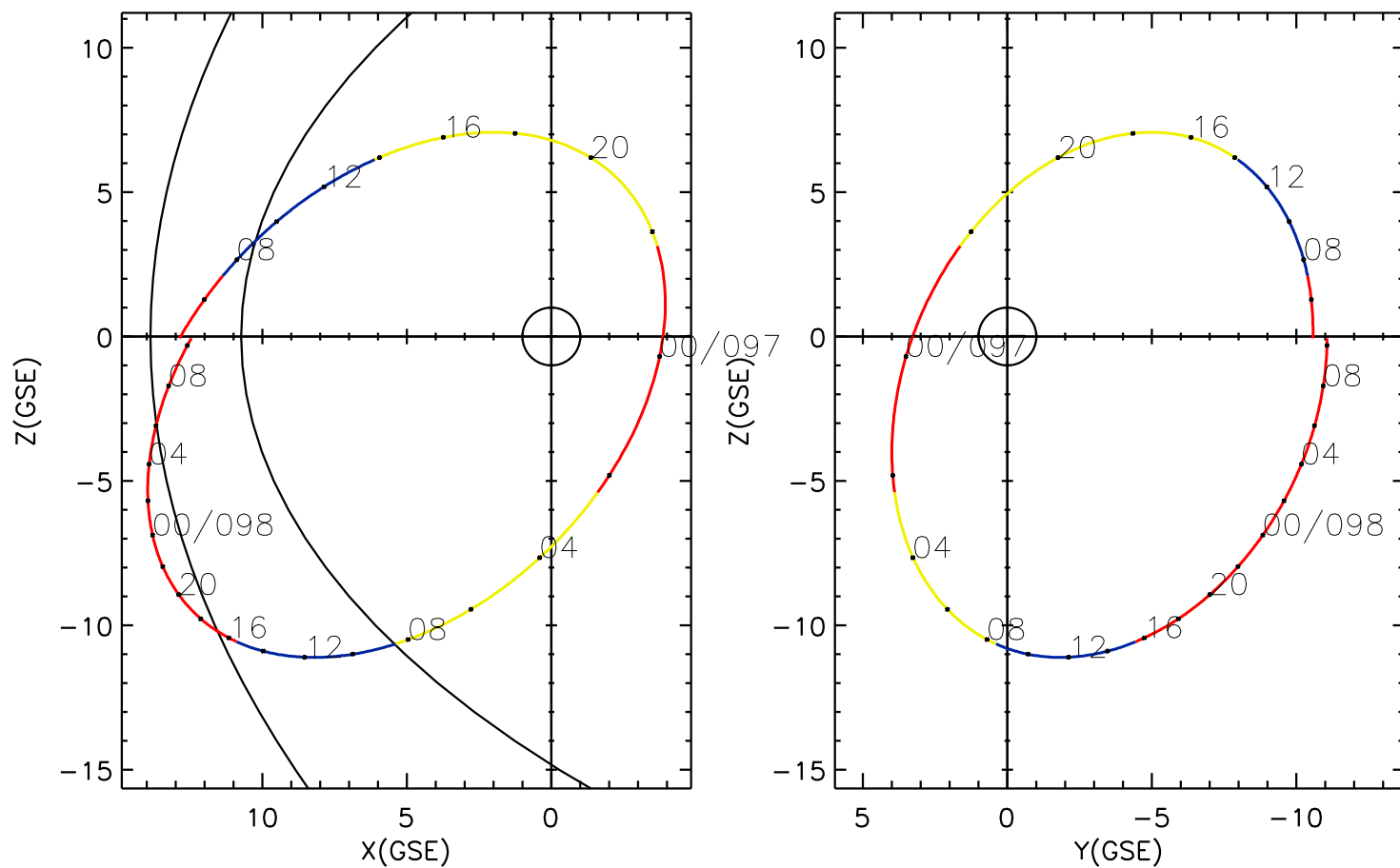
CLUSTER 2 orbit 2016 096 (04/05) 04:06 UT to 2016 098 (04/07) 10:21 UT
