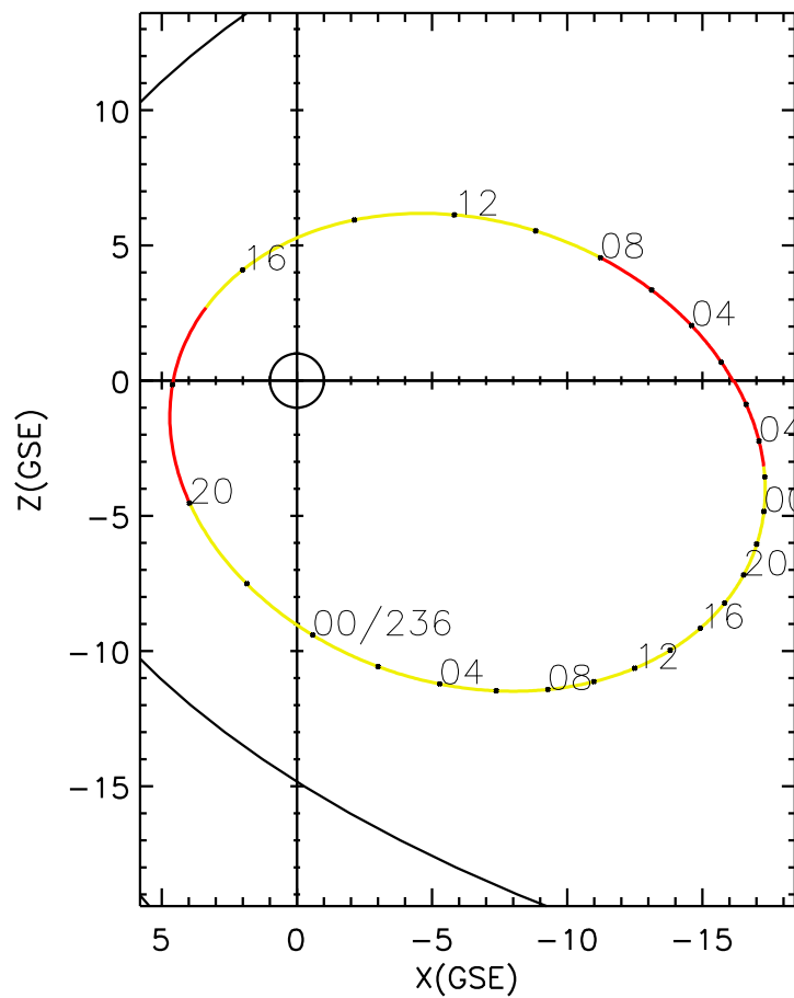
CLUSTER 2 orbit 2015 235 (08/23) 00:56 UT to 2015 237 (08/25) 07:16 UT
