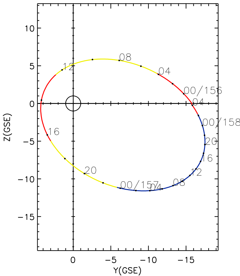
CLUSTER 2 orbit 2015 155 (06/04) 22:01 UT to 2015 158 (06/07) 04:16 UT
