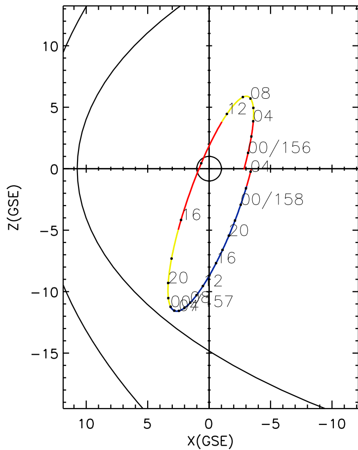
CLUSTER 2 orbit 2015 155 (06/04) 22:01 UT to 2015 158 (06/07) 04:16 UT
