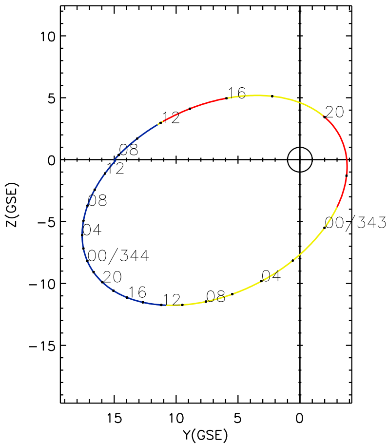
CLUSTER 2 orbit 2014 342 (12/08) 07:21 UT to 2014 344 (12/10) 13:36 UT
