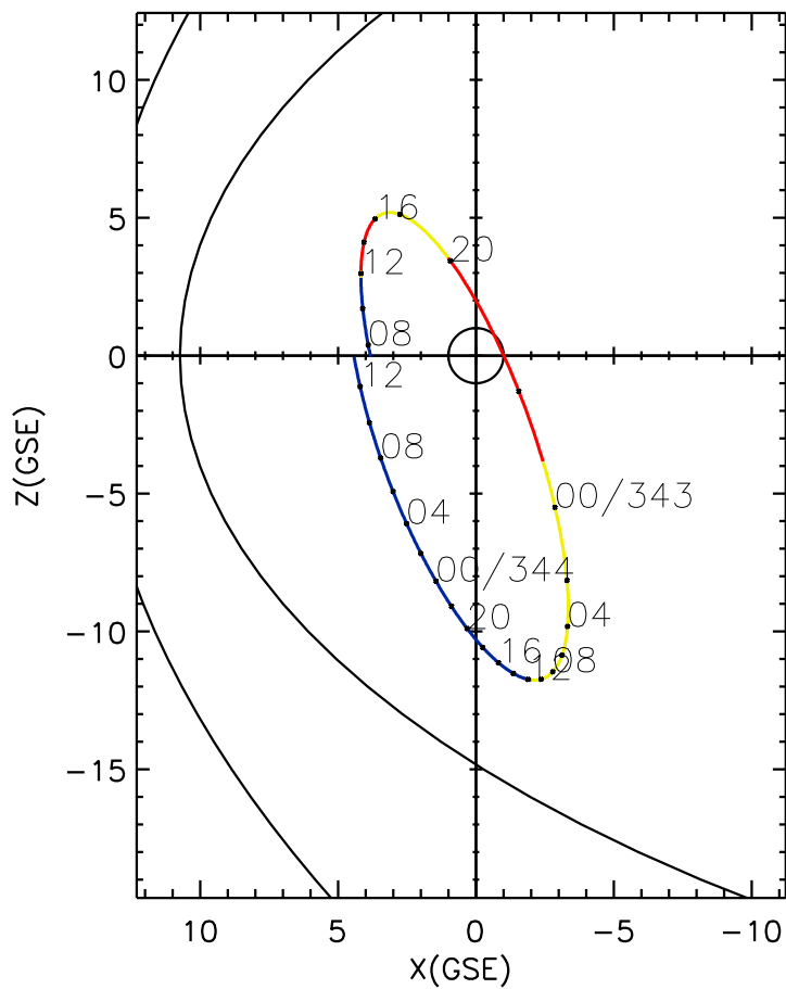
CLUSTER 2 orbit 2014 342 (12/08) 07:21 UT to 2014 344 (12/10) 13:36 UT
