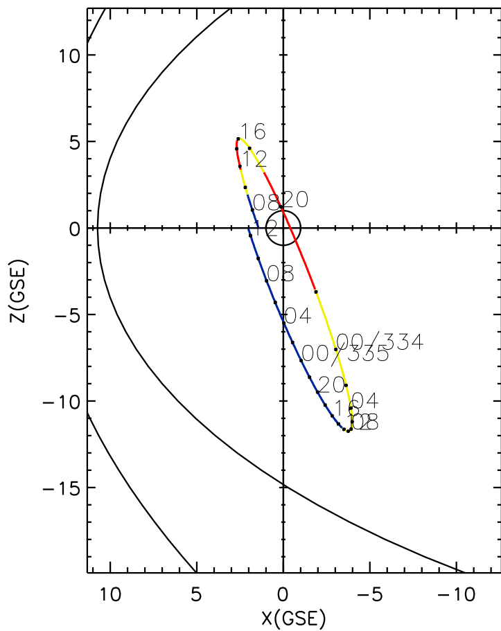
CLUSTER 2 orbit 2014 333 (11/29) 06:21 UT to 2014 335 (12/01) 12:36 UT
