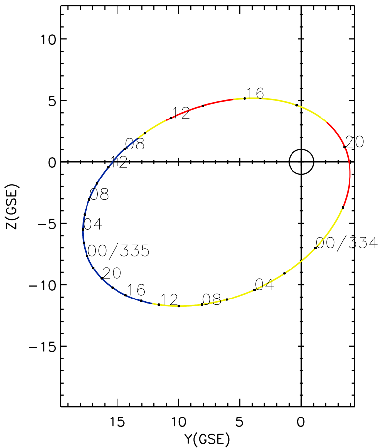
CLUSTER 2 orbit 2014 333 (11/29) 06:21 UT to 2014 335 (12/01) 12:36 UT
