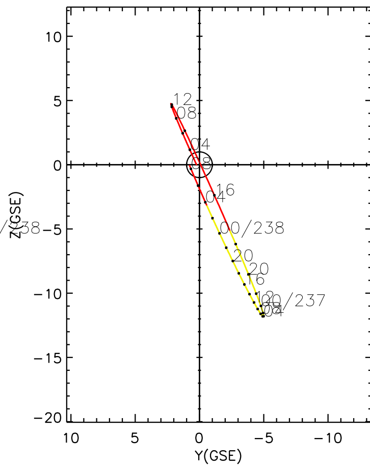
CLUSTER 2 orbit 2014 236 (08/24) 02:11 UT to 2014 238 (08/26) 08:26 UT
