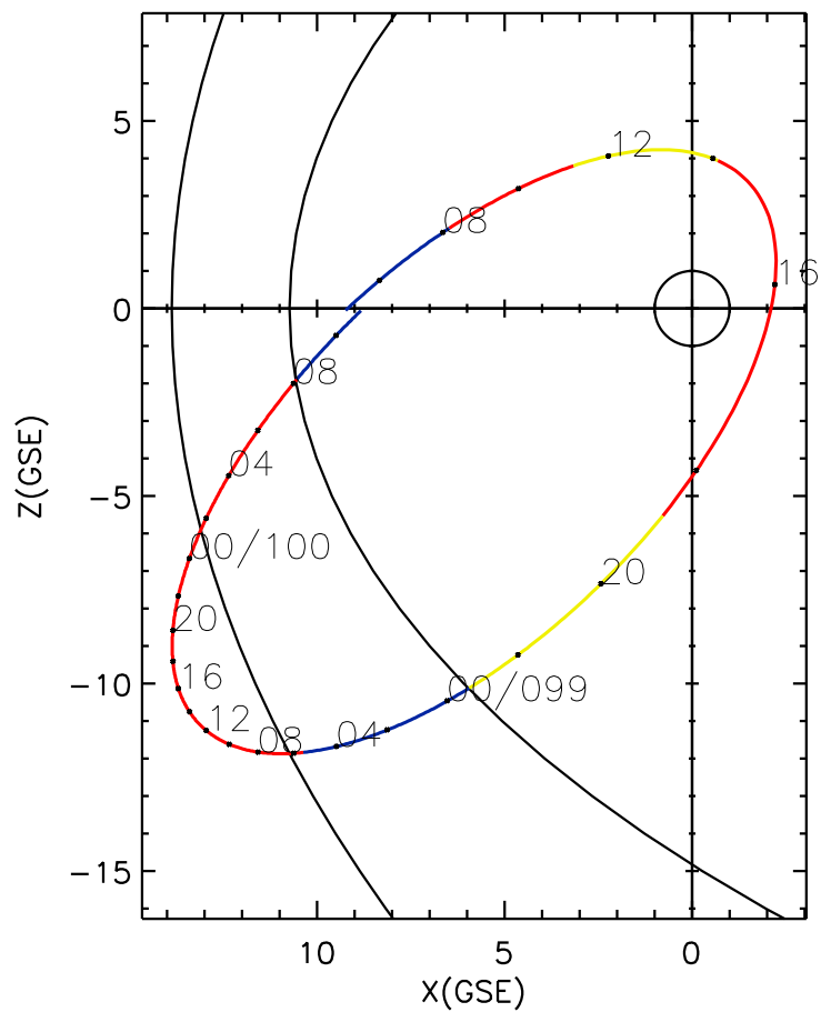
CLUSTER 2 orbit 2014 098 (04/08) 04:46 UT to 2014 100 (04/10) 11:01 UT
