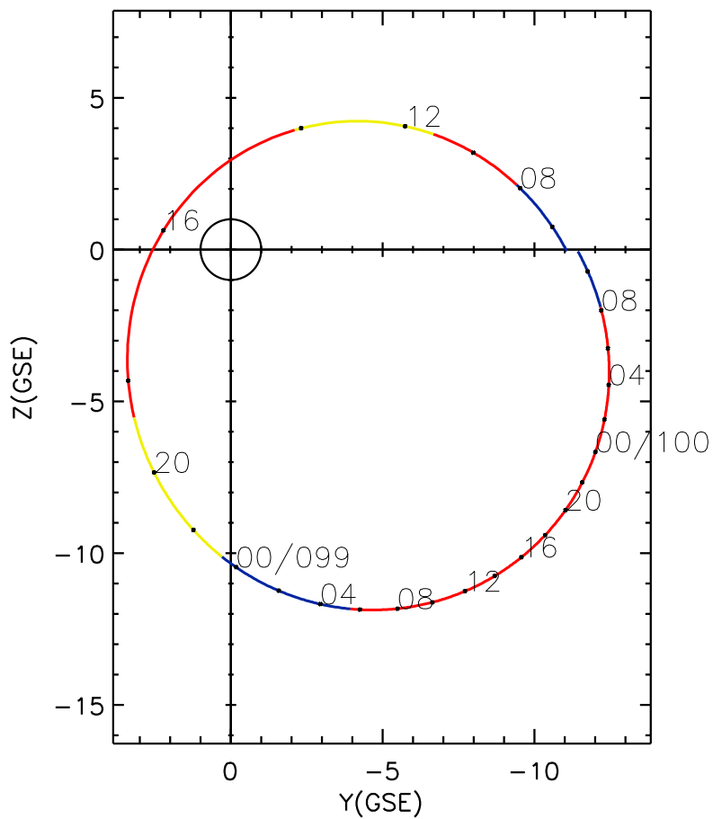
CLUSTER 2 orbit 2014 098 (04/08) 04:46 UT to 2014 100 (04/10) 11:01 UT
