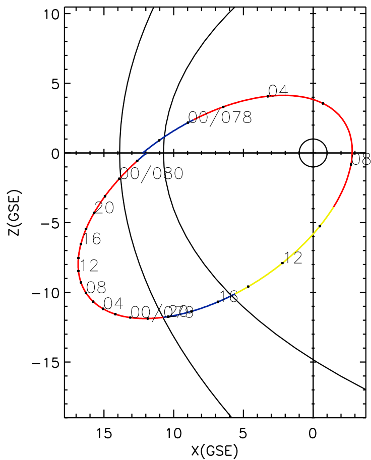
CLUSTER 2 orbit 2014 077 (03/18) 20:36 UT to 2014 080 (03/21) 02:51 UT
