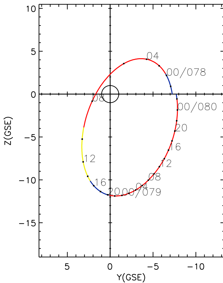
CLUSTER 2 orbit 2014 077 (03/18) 20:36 UT to 2014 080 (03/21) 02:51 UT
