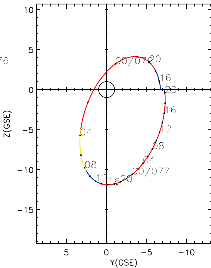
CLUSTER 2 orbit 2014 075 (03/16) 14:21 UT to 2014 077 (03/18) 20:36 UT
