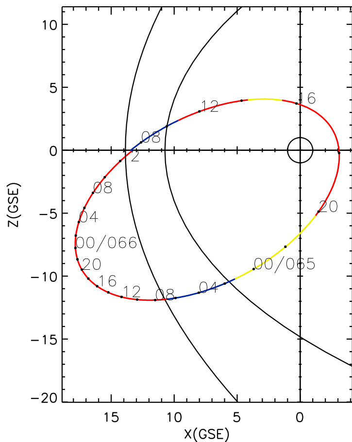
CLUSTER 2 orbit 2014 064 (03/05) 07:01 UT to 2014 066 (03/07) 13:16 UT
