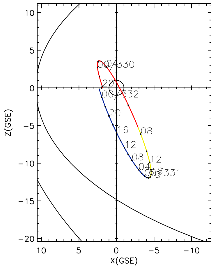
CLUSTER 2 orbit 2013 329 (11/25) 19:36 UT to 2013 332 (11/28) 01:51 UT
