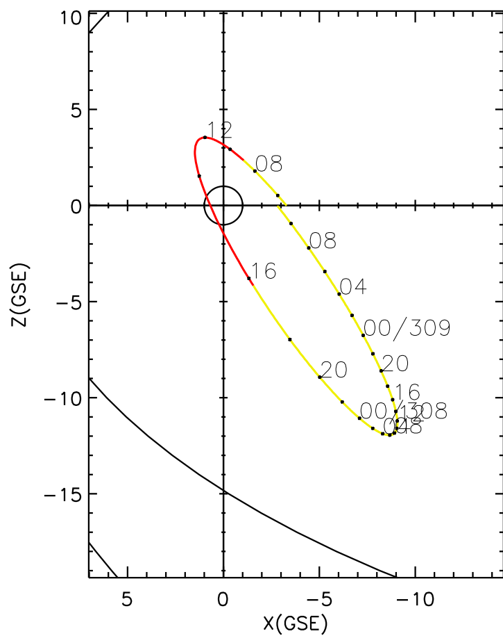
CLUSTER 2 orbit 2013 307 (11/03) 05:11 UT to 2013 309 (11/05) 11:26 UT
