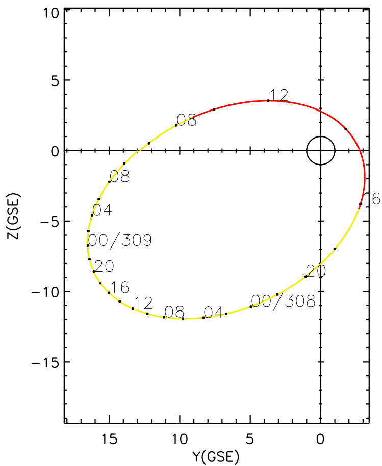
CLUSTER 2 orbit 2013 307 (11/03) 05:11 UT to 2013 309 (11/05) 11:26 UT
