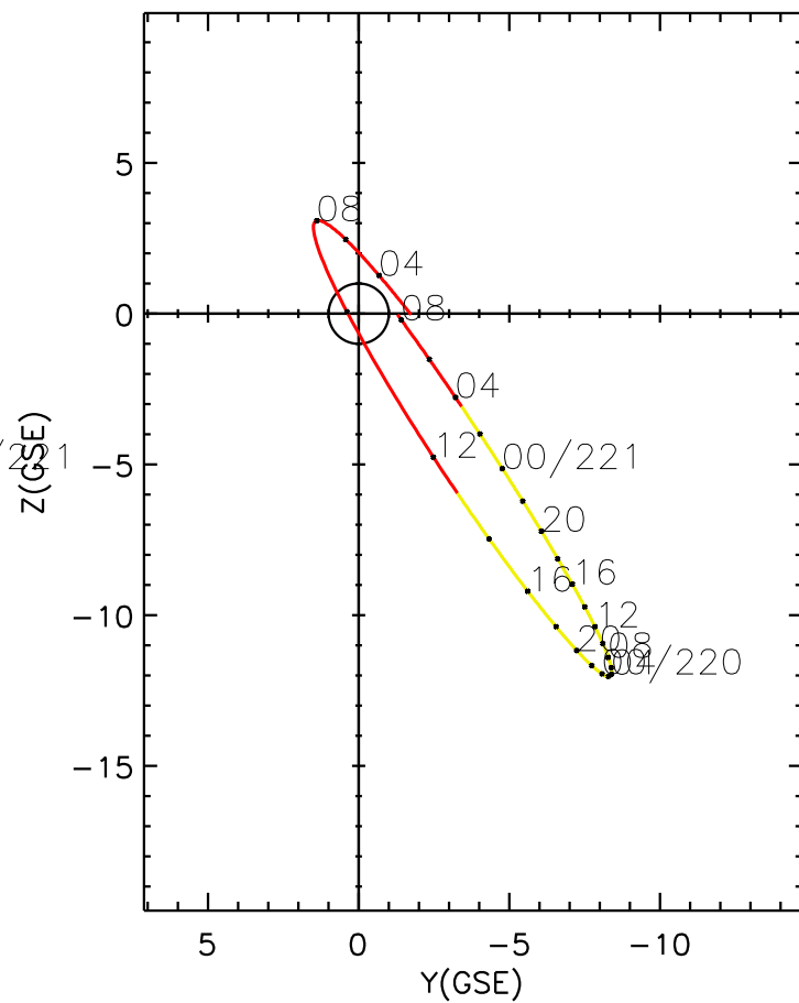
CLUSTER 2 orbit 2013 219 (08/07) 02:01 UT to 2013 221 (08/09) 08:16 UT
