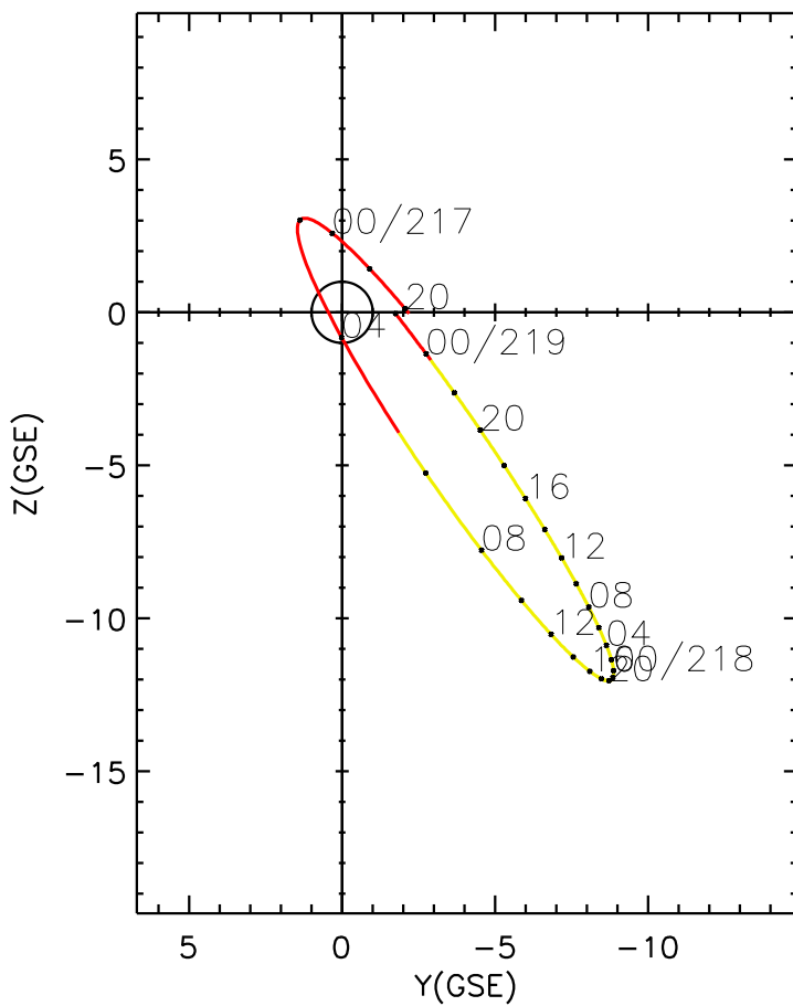
CLUSTER 2 orbit 2013 216 (08/04) 19:46 UT to 2013 219 (08/07) 02:01 UT
