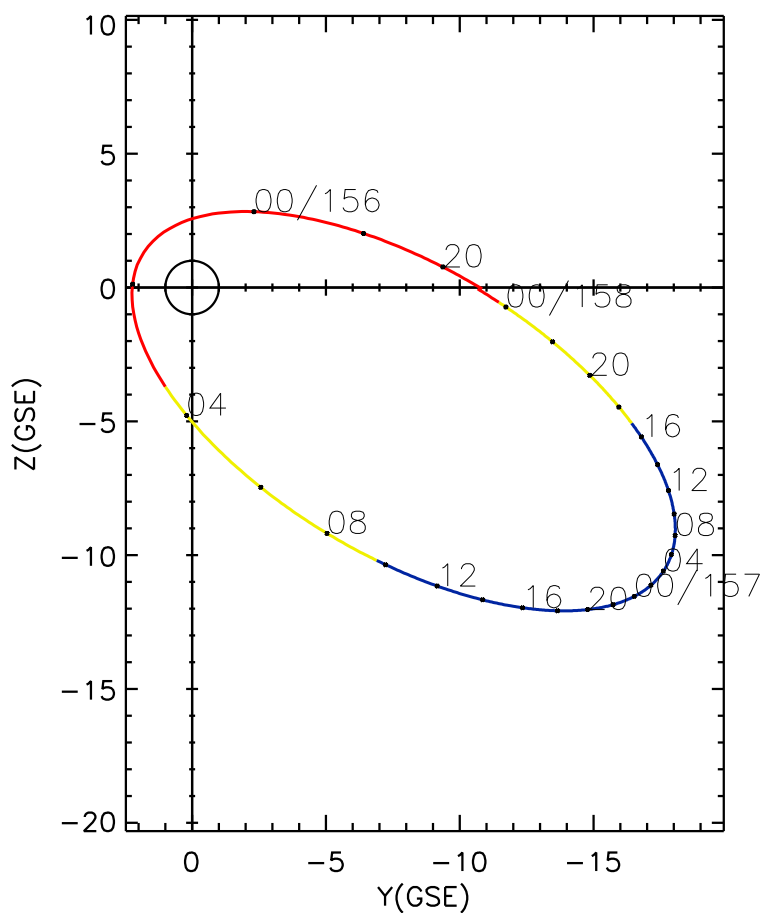
CLUSTER 2 orbit 2013 155 (06/04) 18:46 UT to 2013 158 (06/07) 01:01 UT
