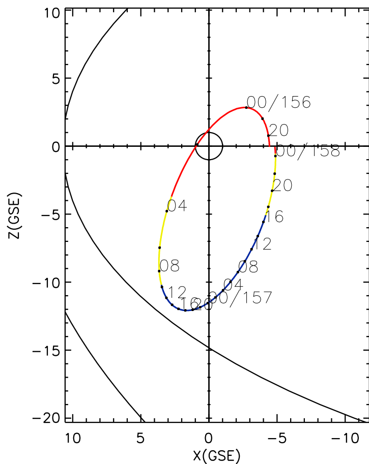
CLUSTER 2 orbit 2013 155 (06/04) 18:46 UT to 2013 158 (06/07) 01:01 UT
