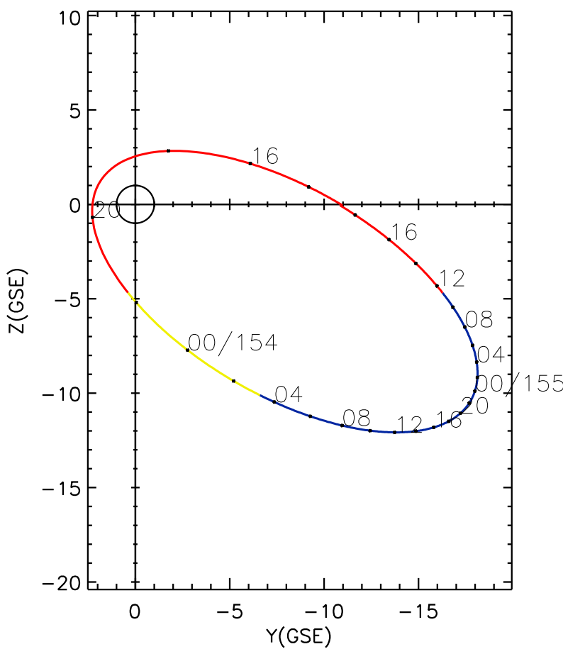
CLUSTER 2 orbit 2013 153 (06/02) 12:31 UT to 2013 155 (06/04) 18:46 UT
