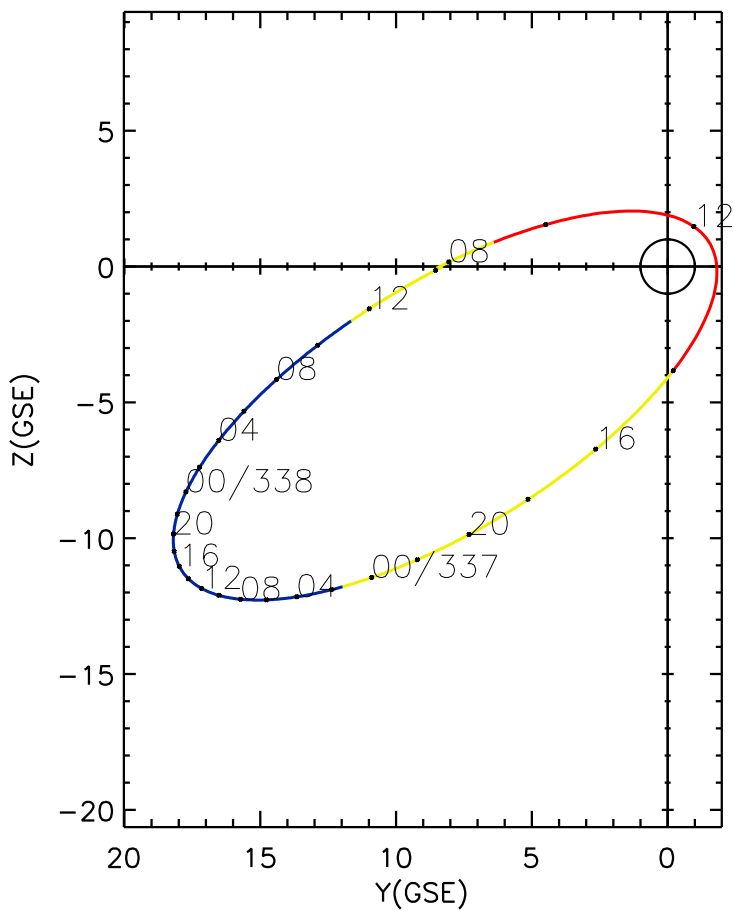
CLUSTER 2 orbit 2012 336 (12/01) 07:41 UT to 2012 338 (12/03) 14:11 UT
