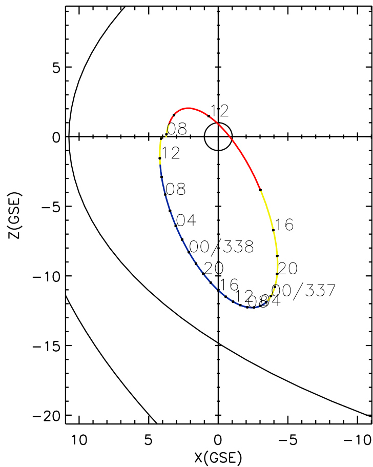
CLUSTER 2 orbit 2012 336 (12/01) 07:41 UT to 2012 338 (12/03) 14:11 UT
