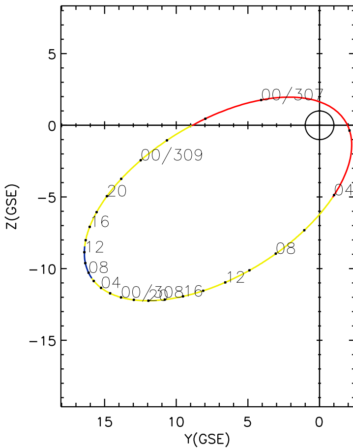
CLUSTER 2 orbit 2012 306 (11/01) 21:21 UT to 2012 309 (11/04) 03:26 UT
