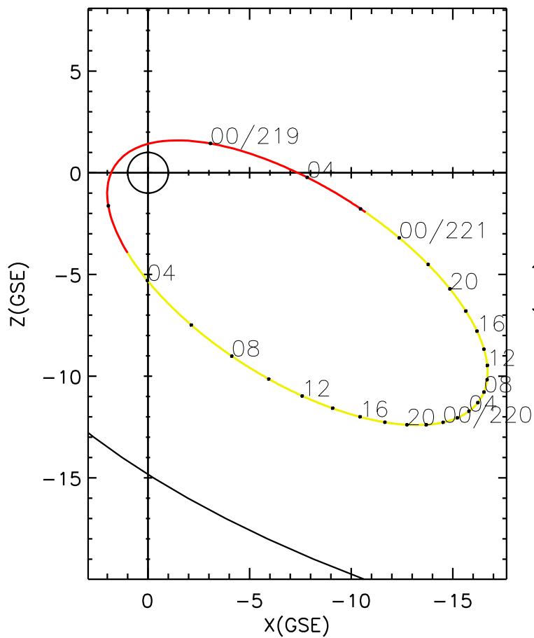
CLUSTER 2 orbit 2012 218 (08/05) 22:01 UT to 2012 221 (08/08) 04:16 UT
