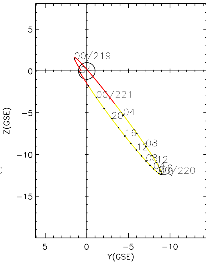
CLUSTER 2 orbit 2012 218 (08/05) 22:01 UT to 2012 221 (08/08) 04:16 UT
