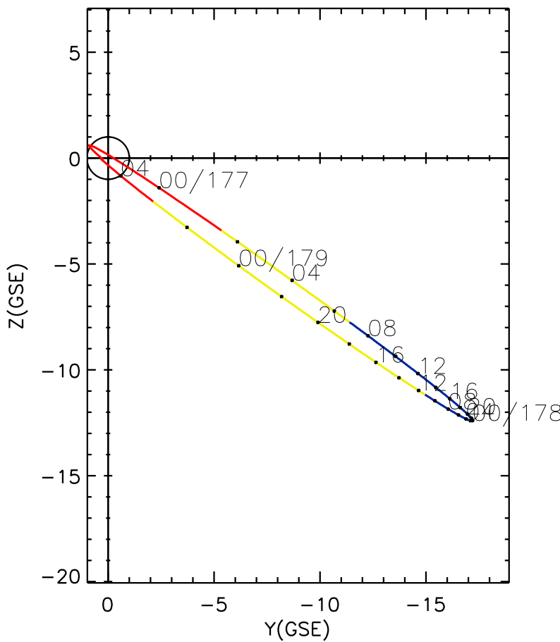
CLUSTER 2 orbit 2011 176 (06/25) 22:16 UT to 2011 179 (06/28) 04:31 UT
