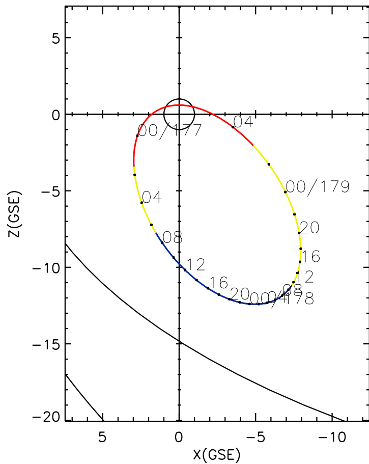
CLUSTER 2 orbit 2011 176 (06/25) 22:16 UT to 2011 179 (06/28) 04:31 UT
