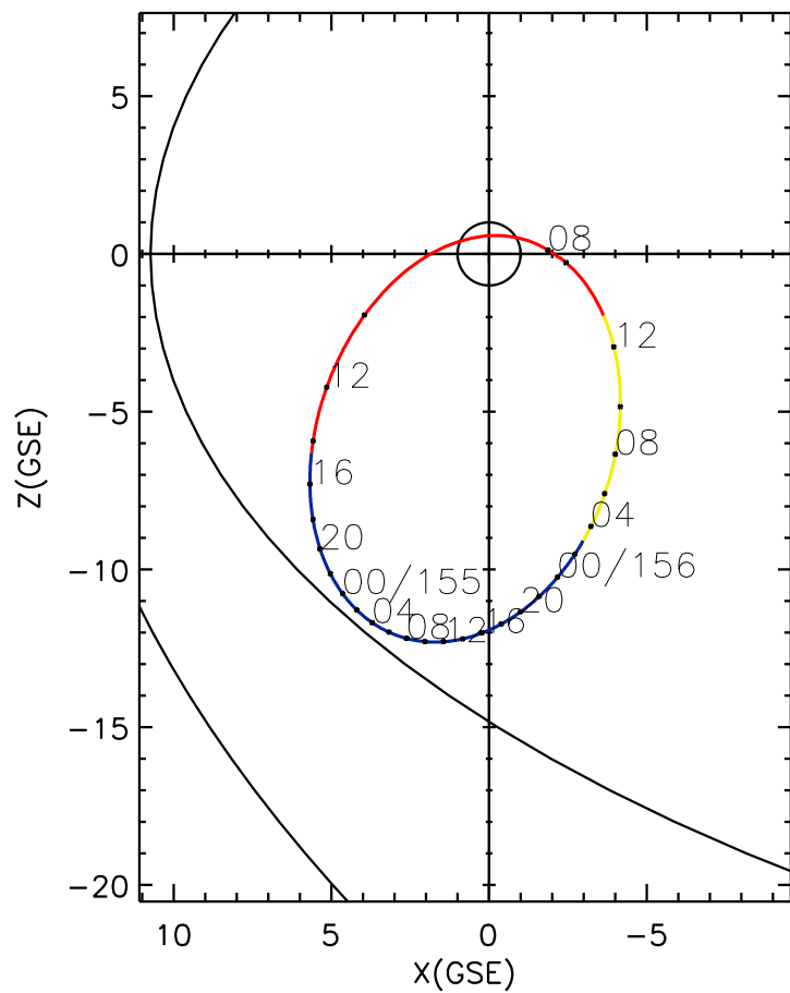
CLUSTER 2 orbit 2011 154 (06/03) 07:51 UT to 2011 156 (06/05) 14:06 UT
