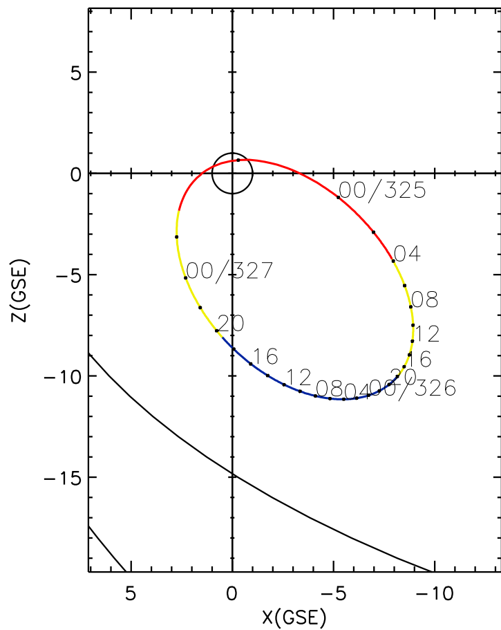
CLUSTER 2 orbit 2010 324 (11/20) 21:36 UT to 2010 327 (11/23) 03:51 UT
