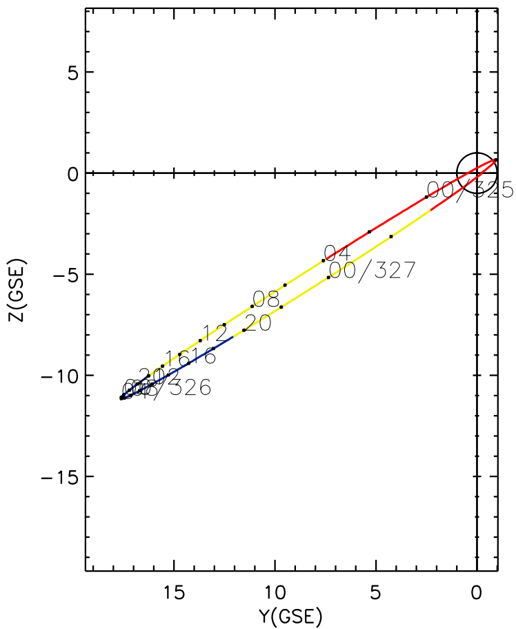
CLUSTER 2 orbit 2010 324 (11/20) 21:36 UT to 2010 327 (11/23) 03:51 UT
