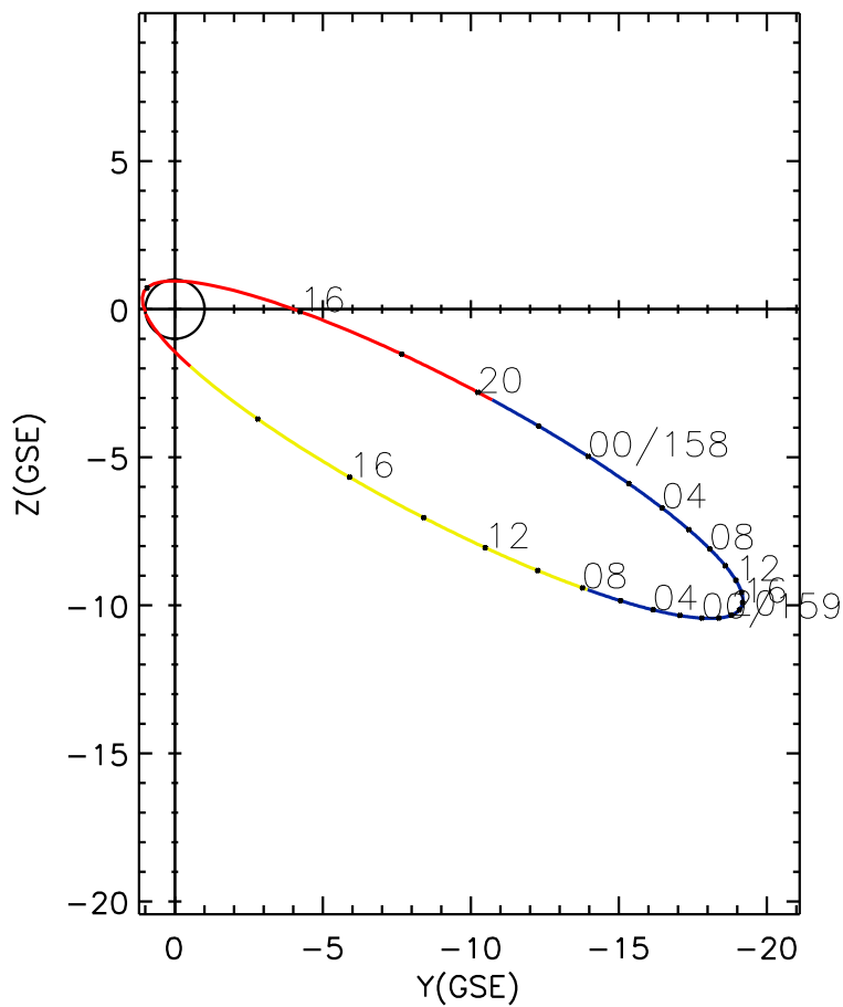
CLUSTER 2 orbit 2010 157 (06/06) 13:41 UT to 2010 159 (06/08) 19:56 UT
