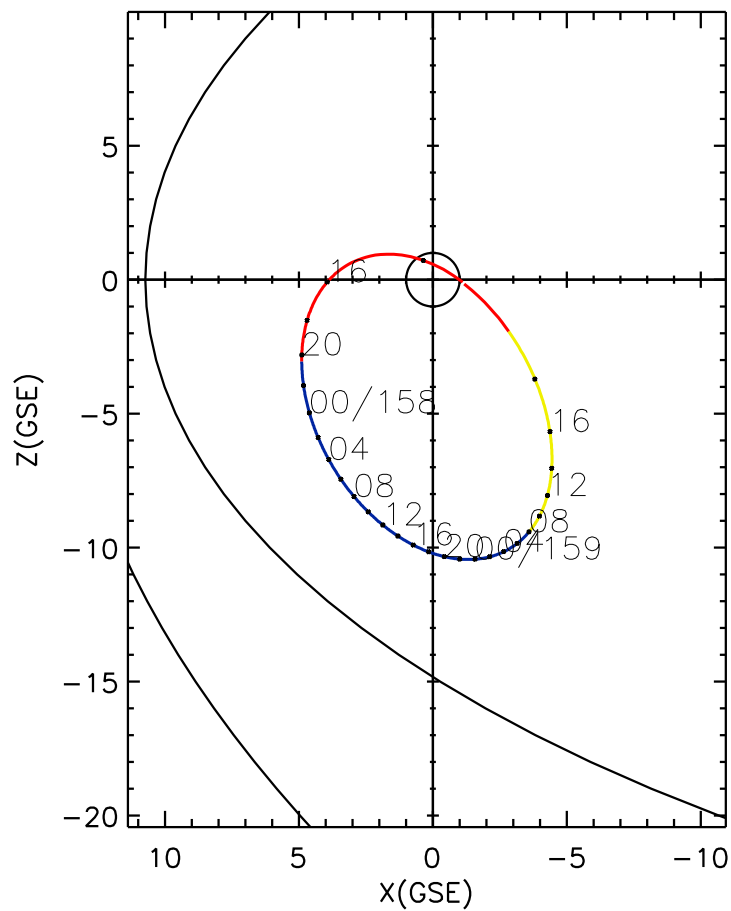
CLUSTER 2 orbit 2010 157 (06/06) 13:41 UT to 2010 159 (06/08) 19:56 UT
