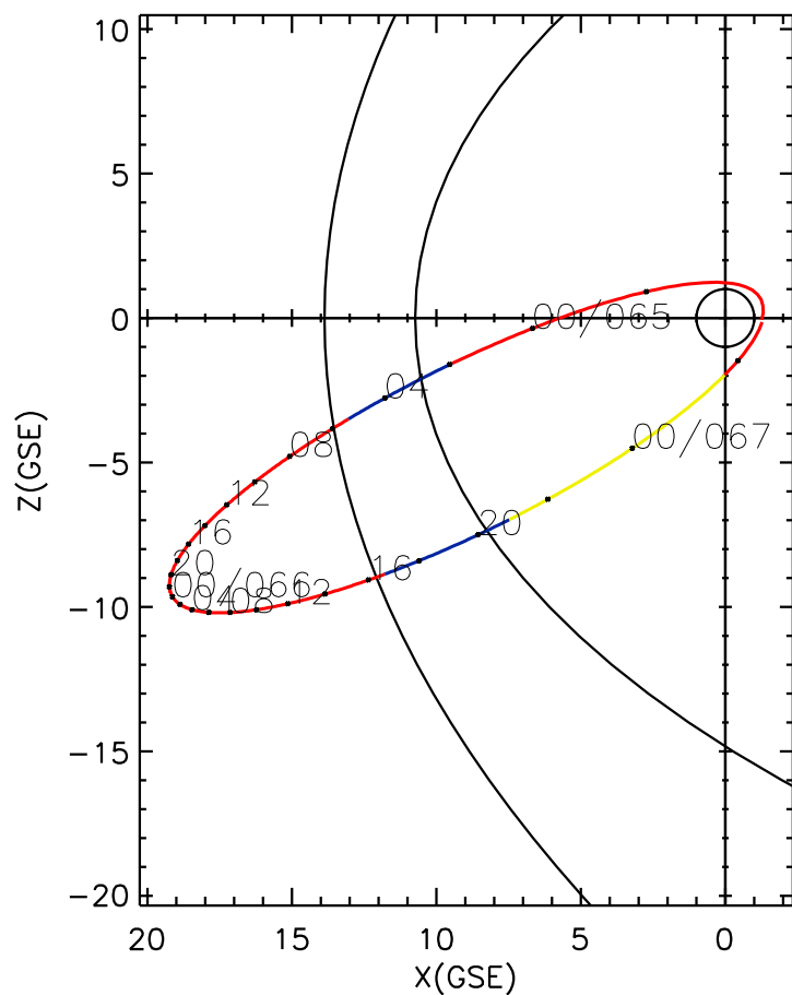
CLUSTER 2 orbit 2010 064 (03/05) 20:16 UT to 2010 067 (03/08) 02:31 UT
