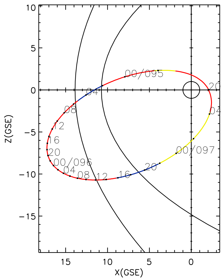
CLUSTER 2 orbit 2009 094 (04/04) 19:56 UT to 2009 097 (04/07) 05:06 UT
