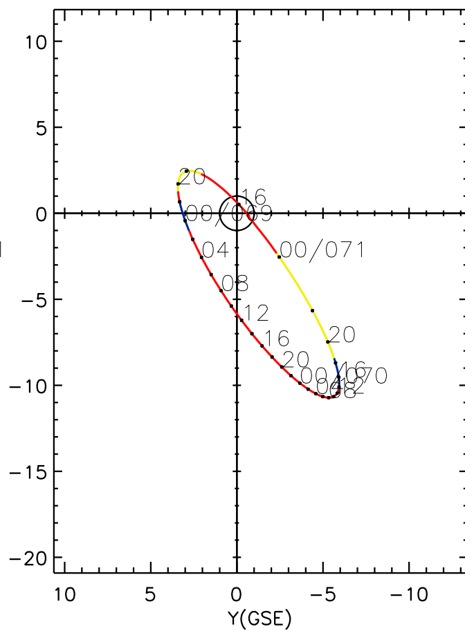
CLUSTER 2 orbit 2009 068 (03/09) 15:46 UT to 2009 071 (03/12) 00:56 UT
