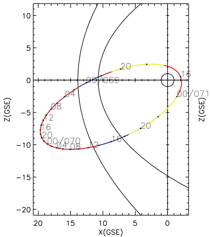
CLUSTER 2 orbit 2009 068 (03/09) 15:46 UT to 2009 071 (03/12) 00:56 UT
