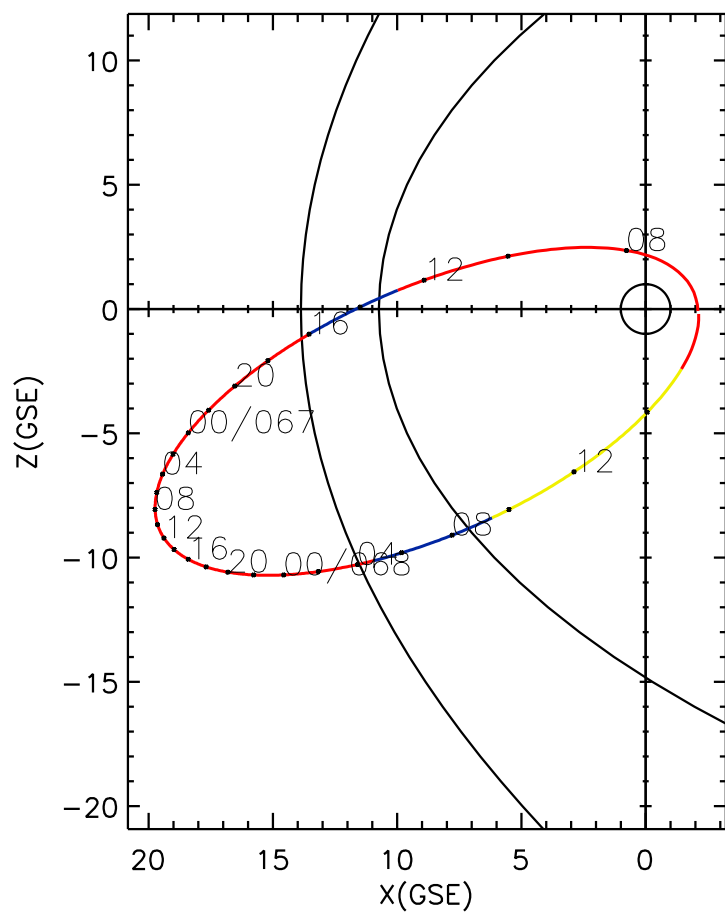
CLUSTER 2 orbit 2009 066 (03/07) 06:41 UT to 2009 068 (03/09) 15:46 UT
