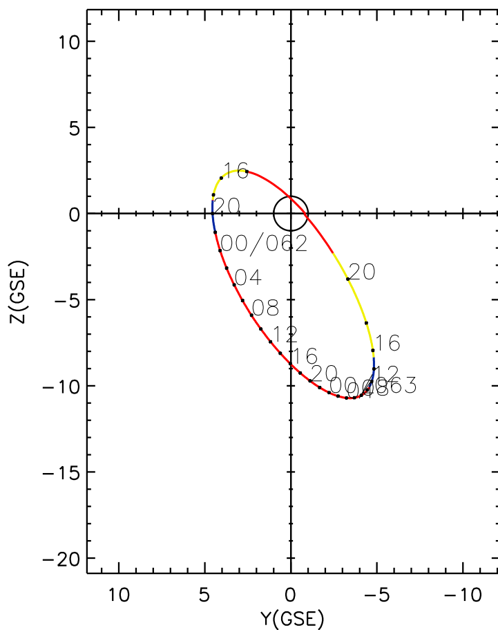
CLUSTER 2 orbit 2009 061 (03/02) 12:31 UT to 2009 063 (03/04) 21:36 UT
