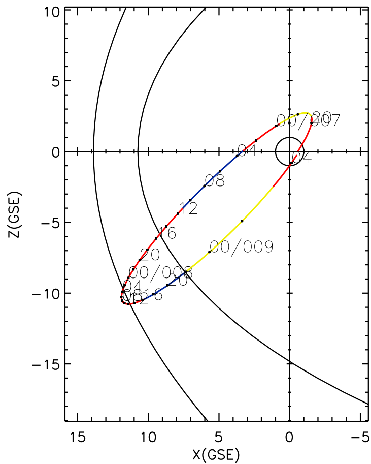
CLUSTER 2 orbit 2009 006 (01/06) 19:11 UT to 2009 009 (01/09) 04:11 UT
