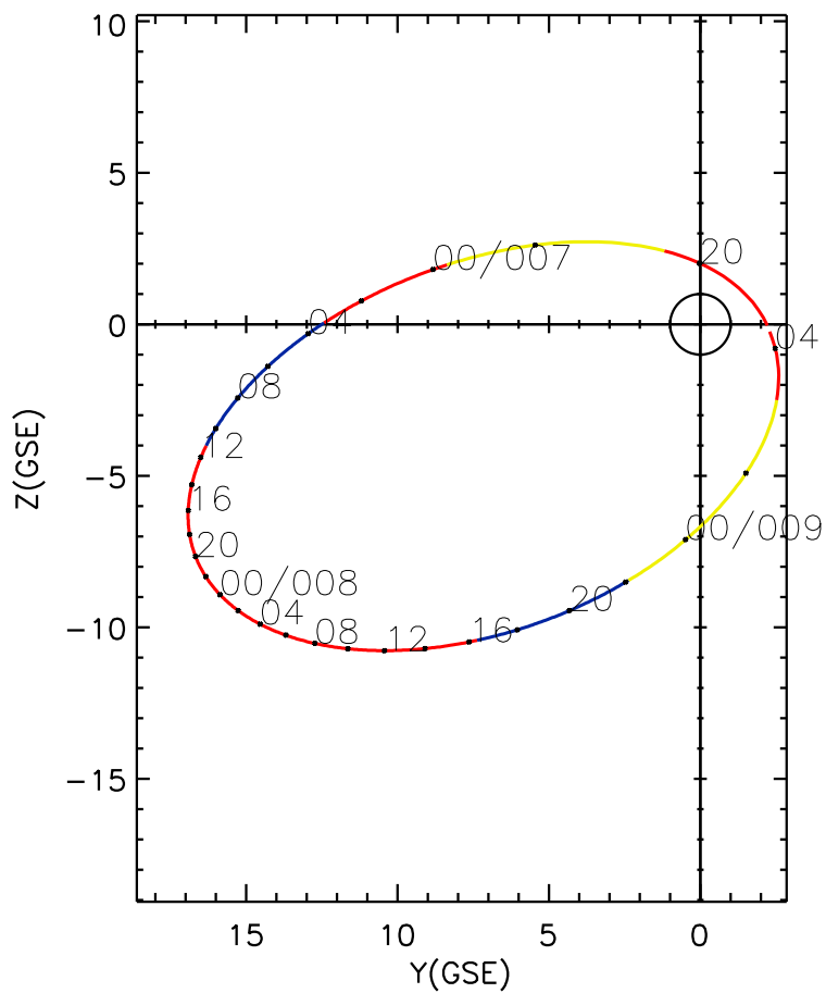
CLUSTER 2 orbit 2009 006 (01/06) 19:11 UT to 2009 009 (01/09) 04:11 UT
