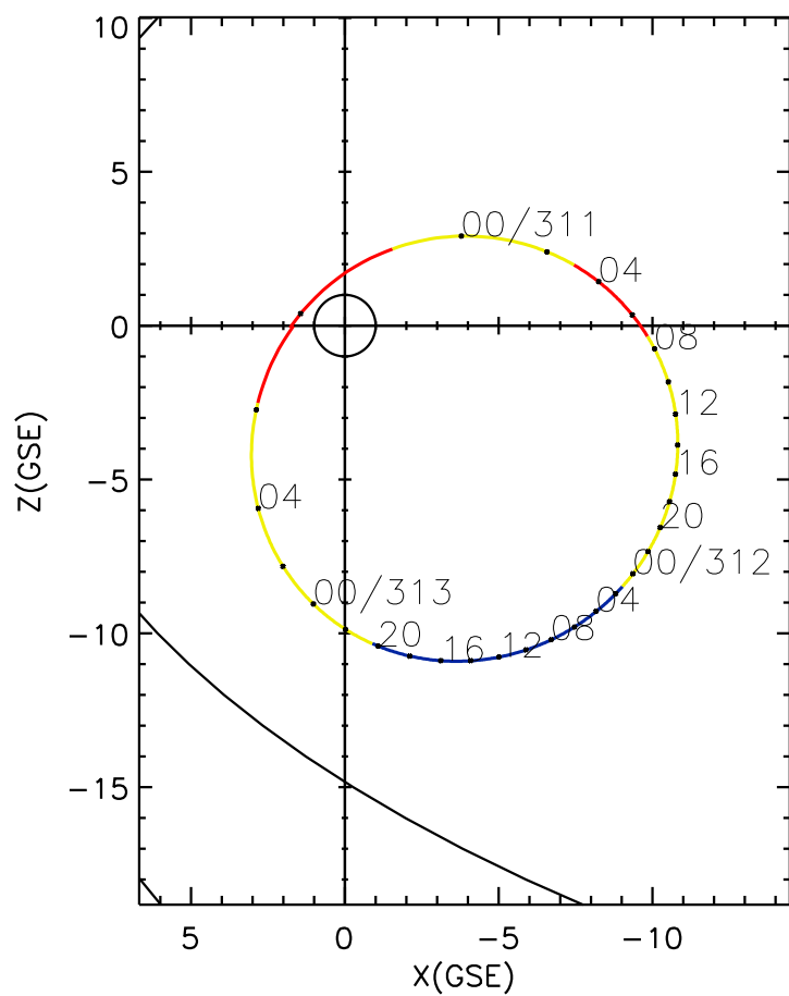
CLUSTER 2 orbit 2008 310 (11/05) 21:51 UT to 2008 313 (11/08) 07:01 UT
