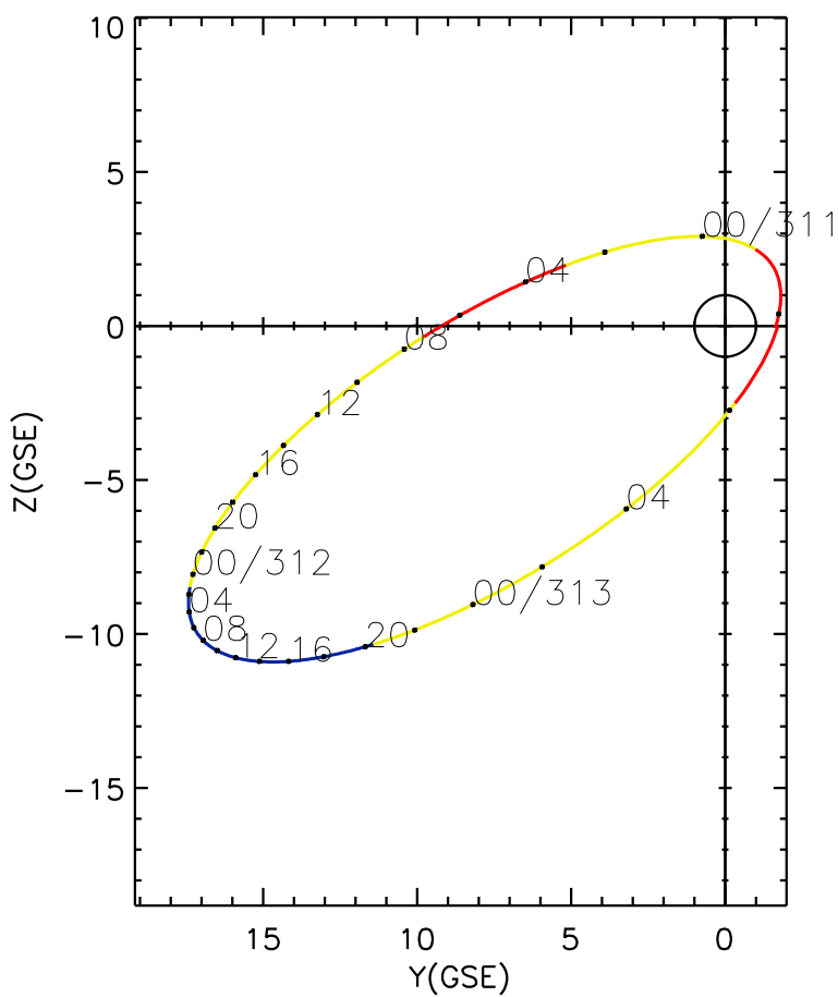
CLUSTER 2 orbit 2008 310 (11/05) 21:51 UT to 2008 313 (11/08) 07:01 UT
