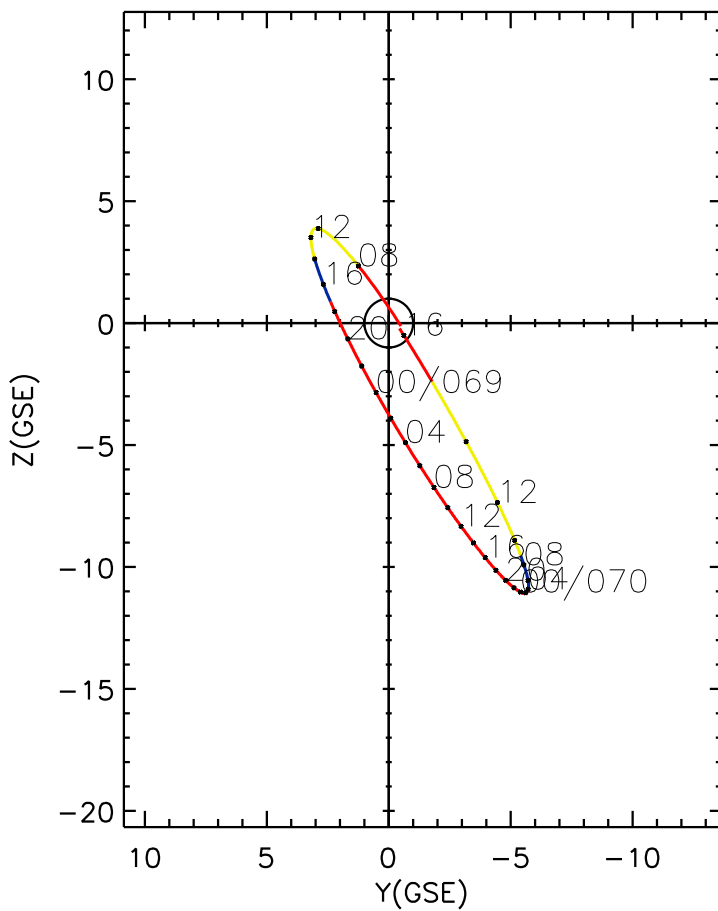
CLUSTER 2 orbit 2008 068 (03/08) 07:01 UT to 2008 070 (03/10) 16:06 UT
