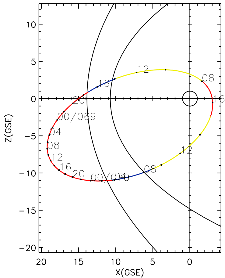
CLUSTER 2 orbit 2008 068 (03/08) 07:01 UT to 2008 070 (03/10) 16:06 UT
