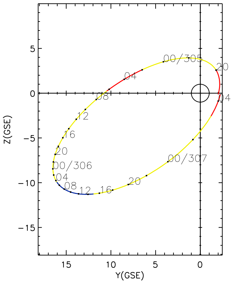
CLUSTER 2 orbit 2007 304 (10/31) 18:56 UT to 2007 307 (11/03) 04:16 UT
