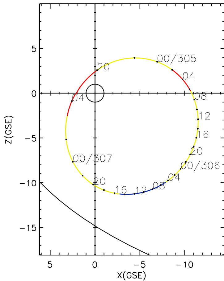
CLUSTER 2 orbit 2007 304 (10/31) 18:56 UT to 2007 307 (11/03) 04:16 UT
