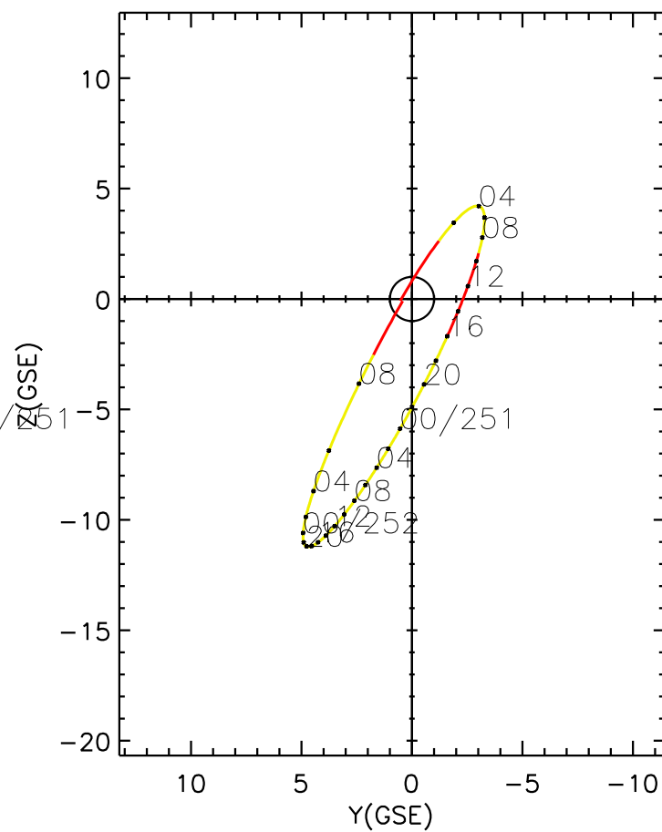
CLUSTER 2 orbit 2007 250 (09/07) 00:21 UT to 2007 252 (09/09) 09:31 UT
