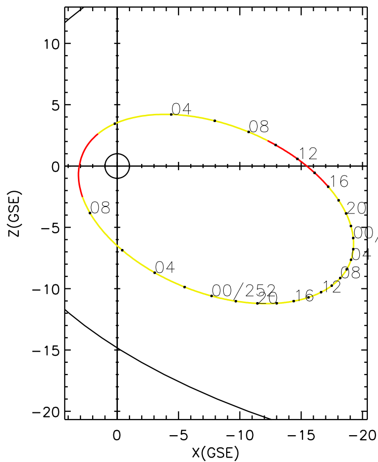
CLUSTER 2 orbit 2007 250 (09/07) 00:21 UT to 2007 252 (09/09) 09:31 UT
